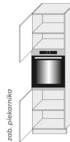
D14 RU 2D 60 (600/2070/565)
