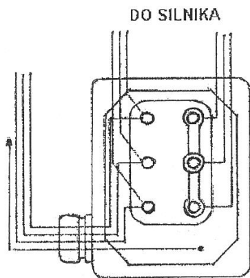
TRZYFAZOWA SIEĆ ELEKTRYCZNA PRĄDU PRZEMIENNEGO
