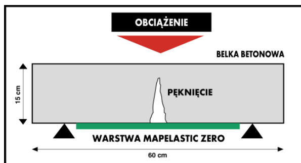
Rys. 1 Wykonanie izolacji Mapelastik Zero na belce betonowej narażonej na działanie obciążeń zginających
