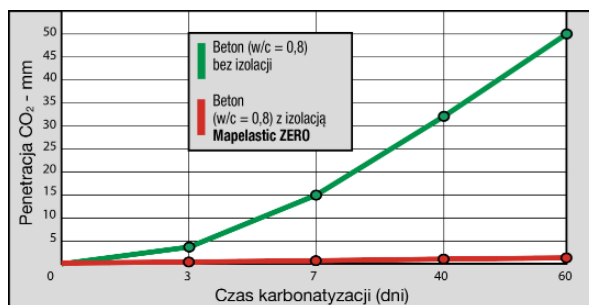
Rys. 2 Wpływ izolacji Mapelastik Zero na ograniczenie karbonatyzacji (30% CO 2 ) w betonie
