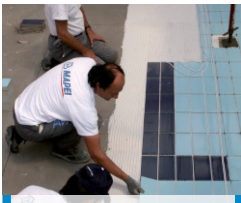
Montaż płytek ceramicznych na warstwie hydroizolacji Mapelastic Zero
