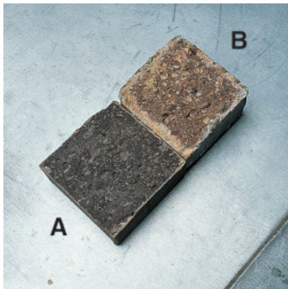
Fot. 2 B - Próba penetracji jonami chloru (UNI 9944). Próbką A została zabezpieczona izolacją Mapelastik Zero i nie wykazuje penetracji; próbką B, bez izolacji wykazuje zniszczenia różnej wielkości
