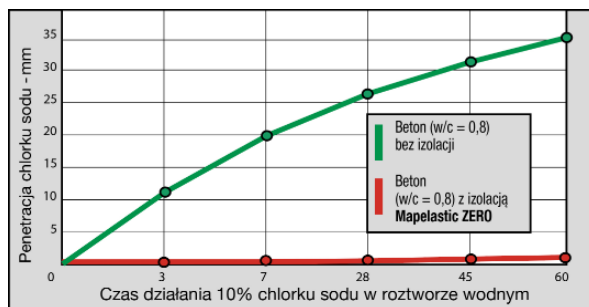
Rys. 3 Wpływ izolacji Mapelastik Zero na ograniczenie penetracji chlorków sodu w porowatym betonie
