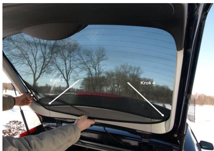
Zdj. 5, 6, 7 – Montaż zasłony klapy bagażnika
