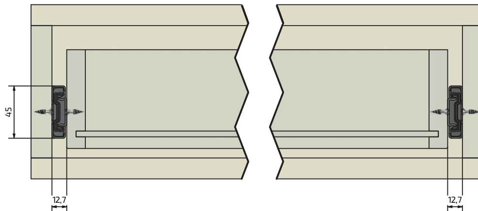
Widok szuflady od boku
