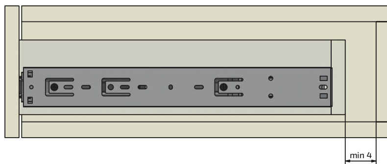
Montaż prowadnic do szuflady i korpusu
