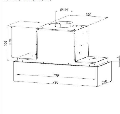
Rys.2: Rysunek gabarytowy
