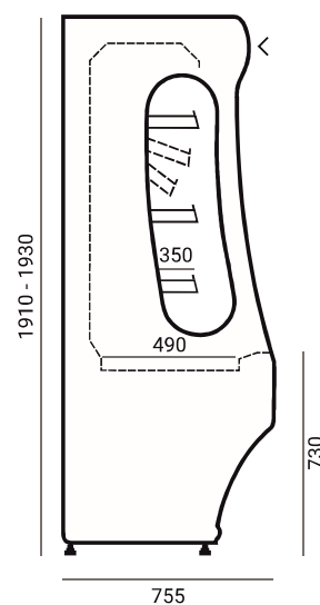
RCh-1/B WERSJA CHŁODNICZA
