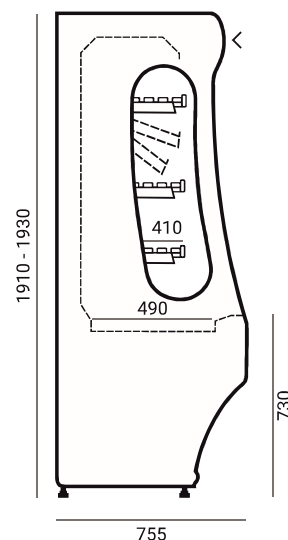
RCh-1/B/W WERSJA CHŁODNICZO - WARZYNNA
