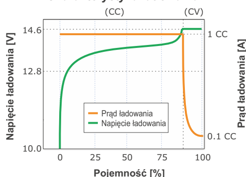
Charakterystyka ładowania
