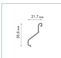
ŁĄCZNIK LK30/LK40
