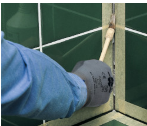
Gruntowanie boków szczeliny przy użyciu Primer FD
