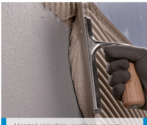
Montaż okładziny podłogowej przy użyciu zaprawy klejącej Keraflex Maxi S1
