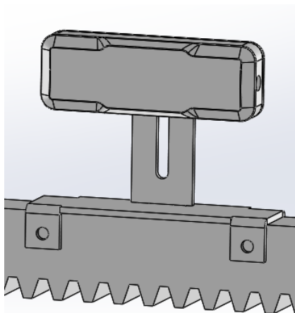
Rys. 7. Wizualizacja instalacji magnetycznych wyłączników krańcowych.
