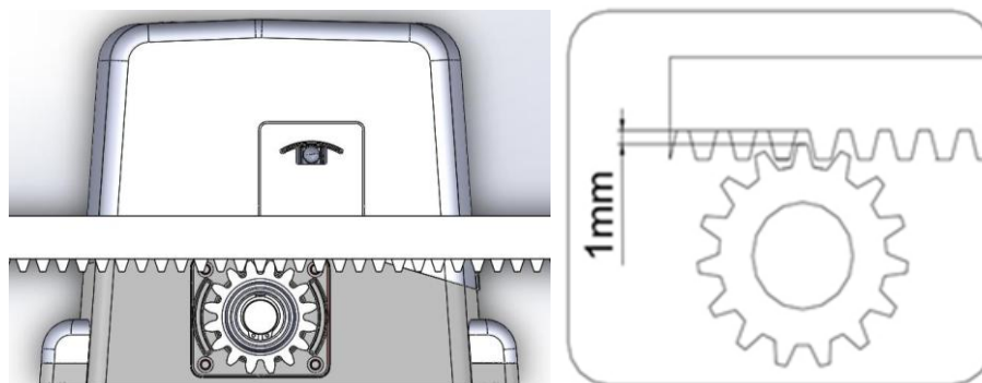
Rys. 3. Dopasowanie koła zębatego do listwy zębatej.
