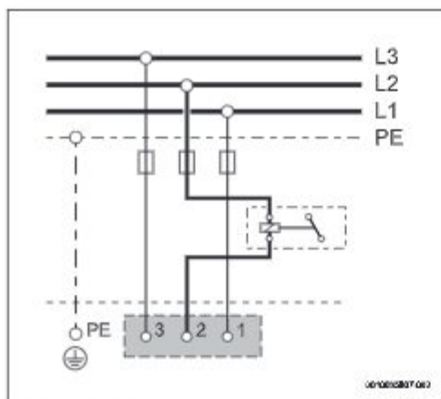
Bild 42 Schaltplan
