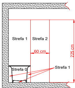
Widok boczny. Wanna
