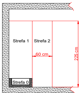
Widok boczny. Prysznic
