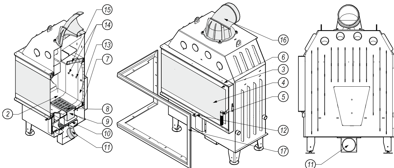
Rysunek 3. Budowa wkładu kominkowego DEFRO HOME PRIMA BL i BP (odbicie lustrzane wersji BL) z drzwiami rozwieralnymi i szybą boczną.
