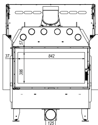
Rysunek 21. Wymiary wkładu kominkowego DEFRO HOME PRIMA LA T.G.
