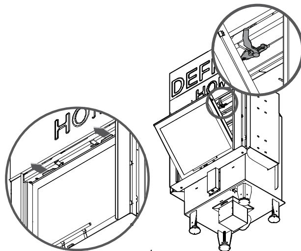
Rysunek 30. Umieszczenie rygli pozwalających na otwarcie drzwi gilotynowych w pozycji uchyłnej wkładu kominkowego DEFRO HOME PRIMA w wersji G.
