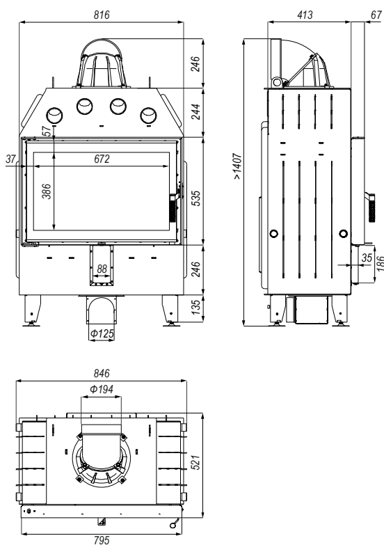
Rysunek 6. Wymiary wkładu kominkowego DEFRO HOME PRIMA ME.
