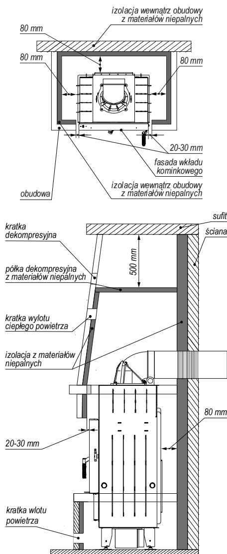
Rysunek 23. Przykładowa zabudowa wkładu kominkowego.
