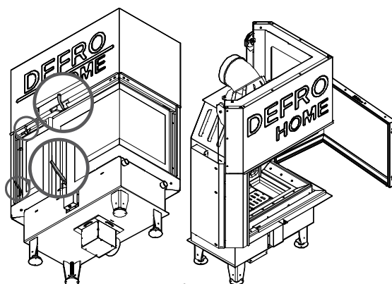
Rysunek 31. Umieszczenie rygli pozwalających na otwarcie drzwi w pozycji uchyłnej w drzwiach gilotynowych z szybą boczną kominka DEFRO HOME PRIMA w wersji BP(BL) G.
