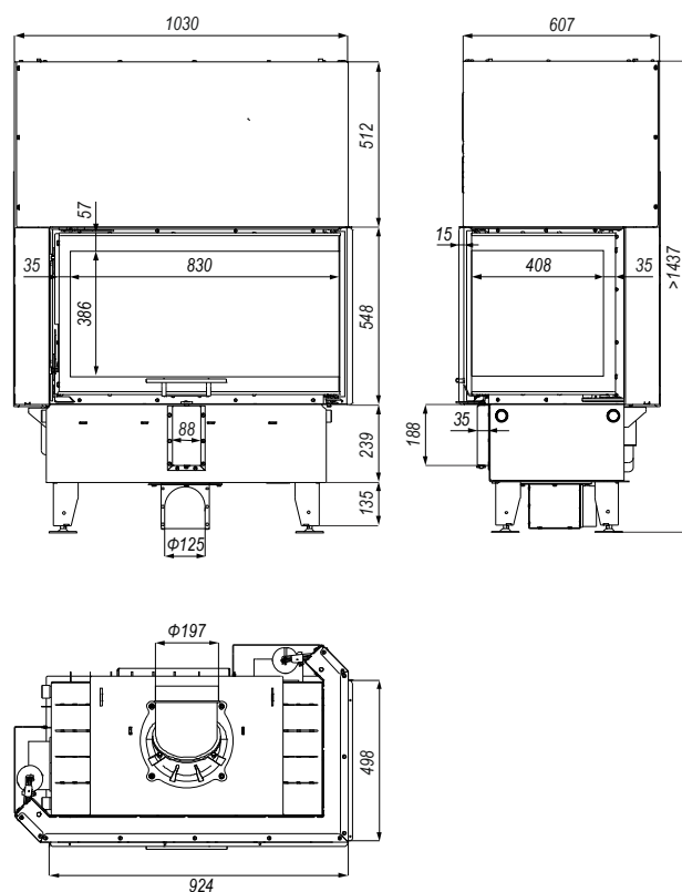
Rysunek 16. Wymiary wkładu kominkowego DEFRO HOME PRIMA ME BP G.
