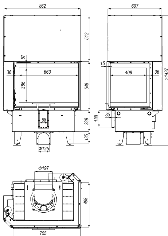
Rysunek 15. Wymiary wkładu kominkowego DEFRO HOME PRIMA SM BP G.
