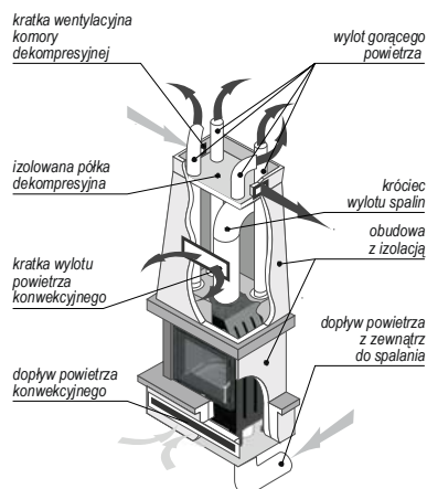
Rysunek 24. System dystrybucji gorącego powietrza.
