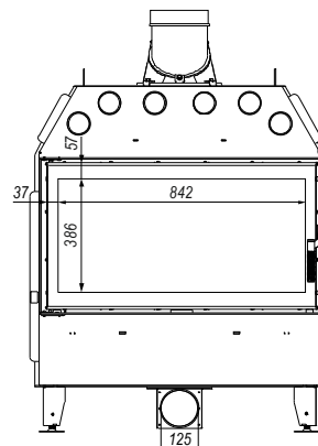
Rysunek 22. Wymiary wkładu kominkowego DEFRO HOME PRIMA LA T.
