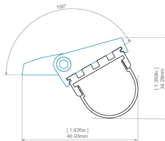
GIZA profile with G-L cover and REGIP-UV mounting bracket profil GIZA z osłoną G-L oraz mocownikiem REGIP-UV
