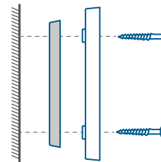
MONTAJE Cuña de montaje
