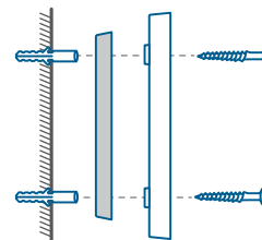
MONTAJE Cuña de montaje
