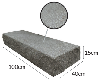
POWIERZCHNIA GŁADKA
