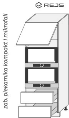
D14 RU 2R KOMPAKT (600/2070/565)
