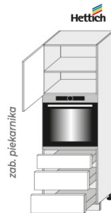
D14 RU 3A 60 (600/2070/565)
