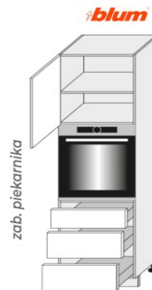
D14 RU 3M 60 ● (600/2070/565)
