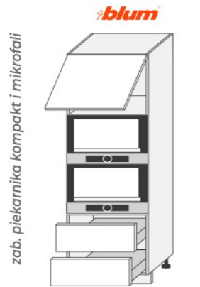
D14 RU 2M KOMPAKT ● (600/2070/565)
