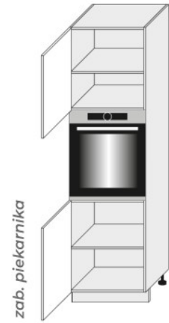
D14 RU 2D 60 (600/2070/565)
