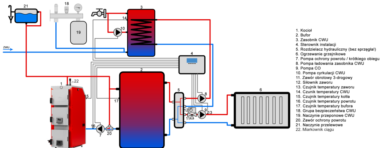
Rysunek nr 4 Schemat instalacji grzewczej zalecany przez producenta
