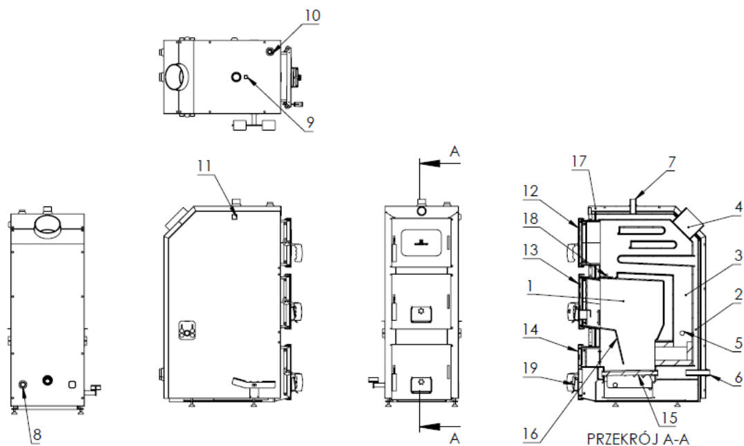
Rysunek nr 2. Budowa kotłów „DrewKo”
