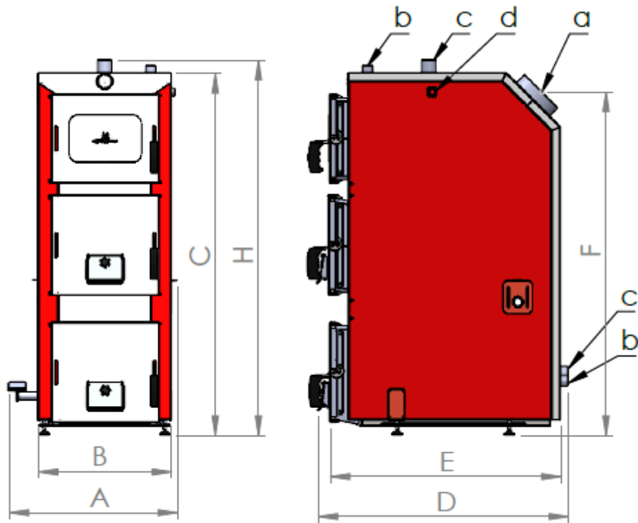
Rysunek nr 1. Wymiary kotłów „DrewKo”
