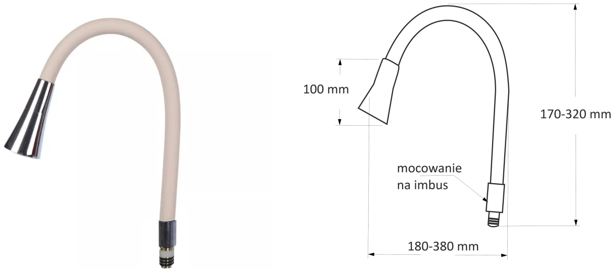
rysunek techniczny
