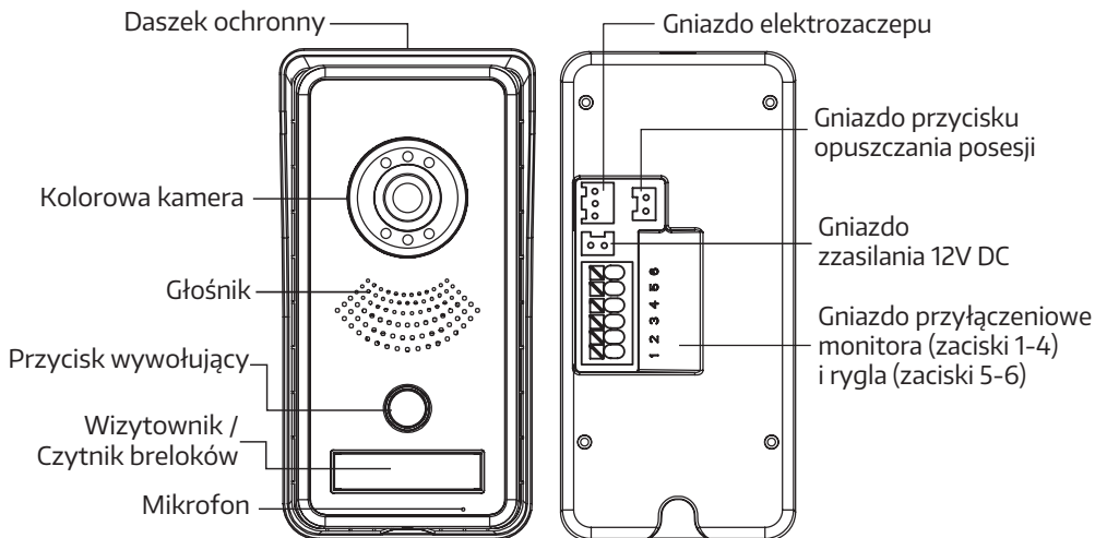
Rys. 1. Budowa kasety VDC-60RU
