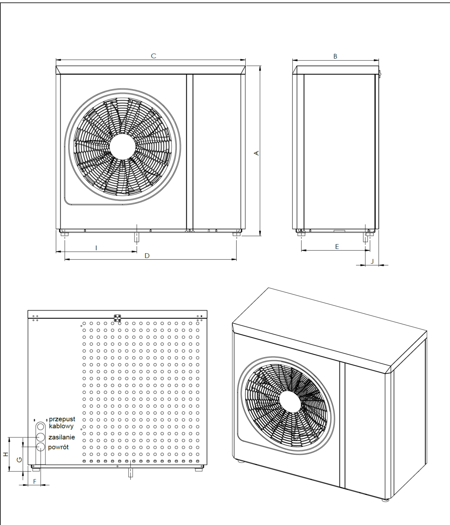
Rysunek 4. Wymiary pomp ciepła AirAdapt wraz z odpływem skroplin i postumentem [mm].
