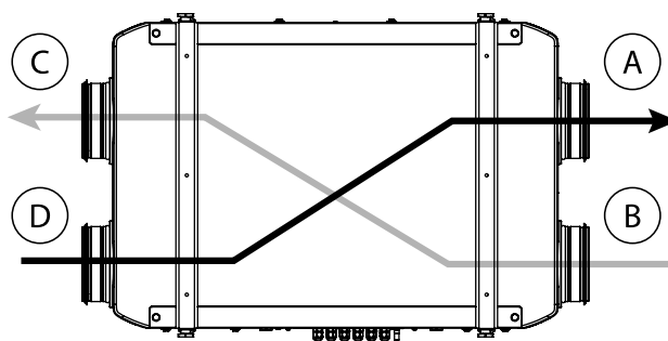
A – wyrzutnia, B – czerpnia, C – nawiew, D – wywiew
