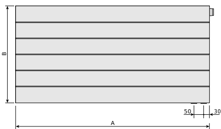
Ramo Ventil Compact, prawy, widok z przodu
