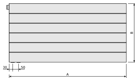
Ramo Ventil Compact, lewy, widok z przodu
