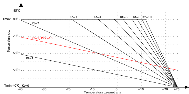
Rys.2.4.2.1 Wykres krzywych grzewczych (ogrzewanie tradycyjne)
