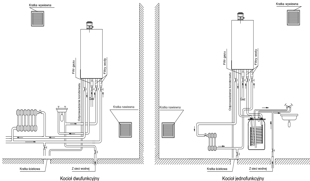
Rys. 3.5.1 Wymagania instalacyjne kotłów
