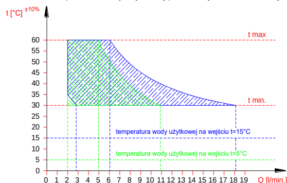
Rys. 2.4.3.1. Wykres temperatury wody użytkowej na wyjściu z kotła typ 20kW w zależności od wielkości przepływu wody.
