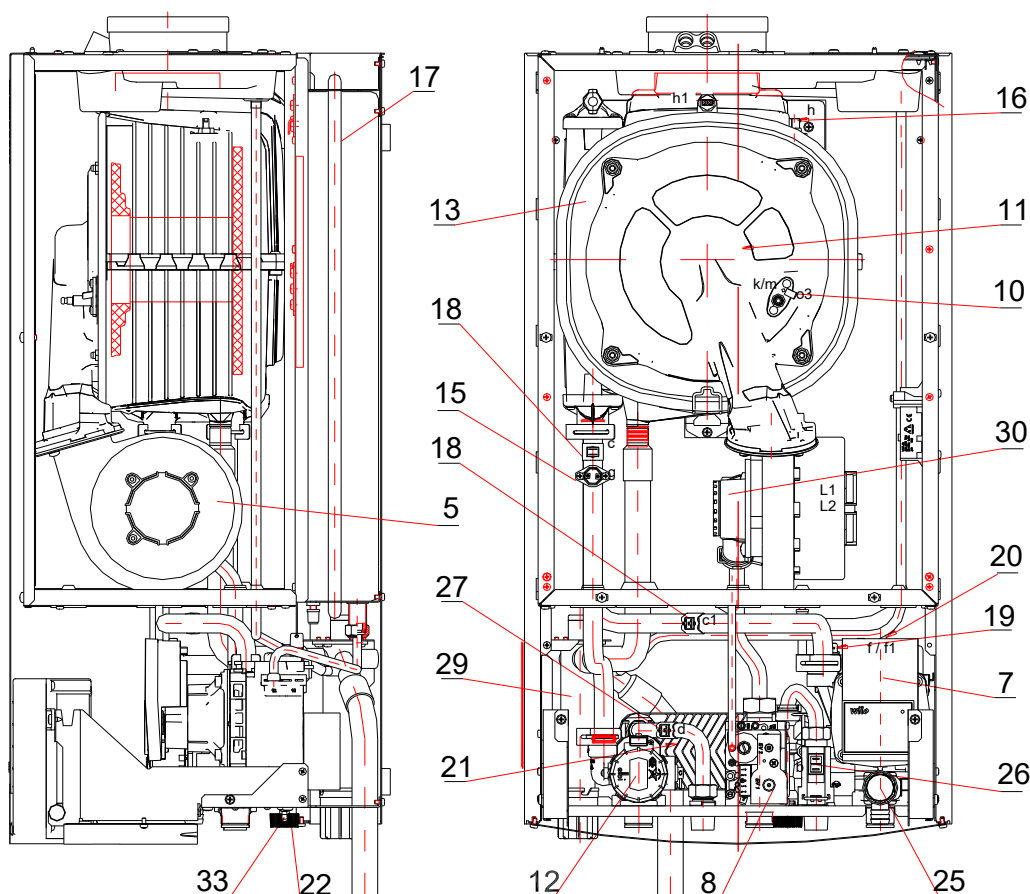
Rys.2.2.1.1. Rozłożenie elementów w kotle ECOCONDENS GOLD PLUS dwufunkcyjnym
