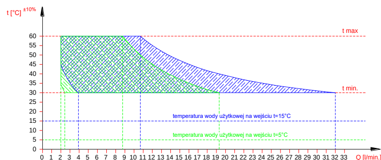
Rys. 2.4.3.3. Wykres temperatury wody użytkowej na wyjściu z kotła typ 35kW w zależności od wielkości przepływu wody.
