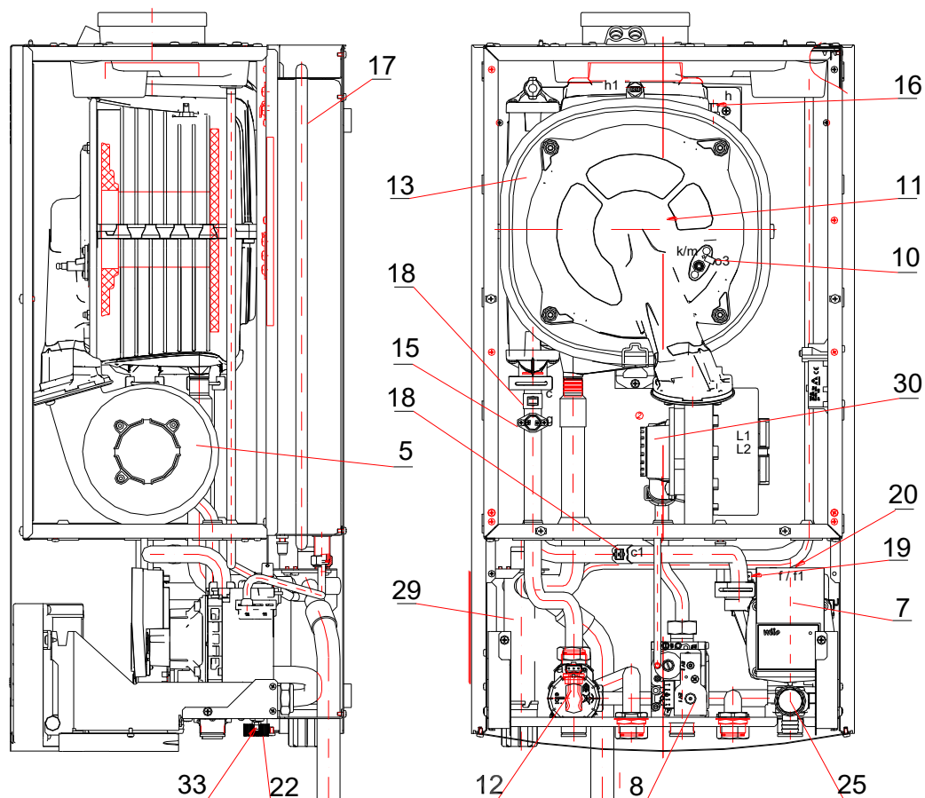
Rys.2.2.1.2. Rozłożenie elementów w kotle ECOCONDENS GOLD PLUS jednofunkcyjnym
