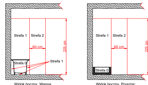
Rys. 3.1.2.1. Wymiary stref w pomieszczeniach zawierających wannę lub prysznic z basenem
