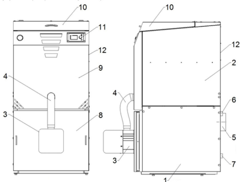
Rys.4. Kocioł „SlimKo Plus”
