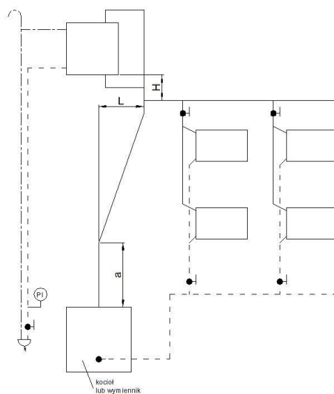
Wariant 1 - rozdziel górny
