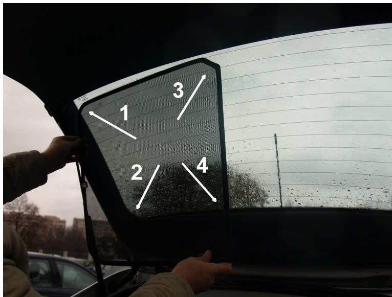
Rys.7 - Montaż zasłonek klapy bagażnika
