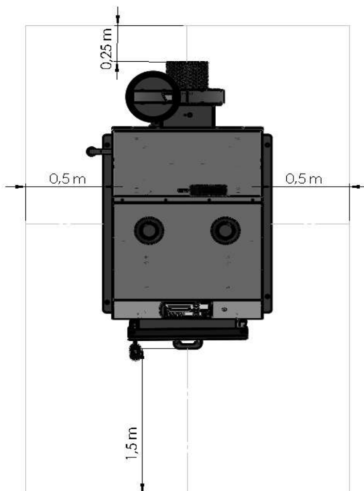
Rys.2 Usytuowanie kotła
