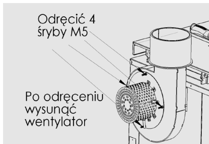
Rys. 11 Czyszczenie dymnicy.
