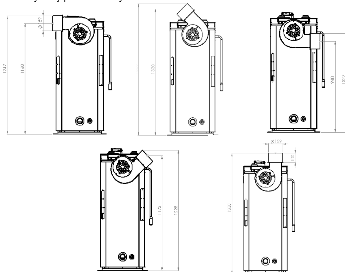
Rys. 3 Konfiguracje dymnicy
