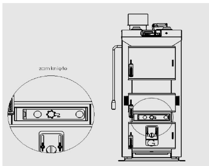
Rys. 10 Regulacja powietrza wtórnego
