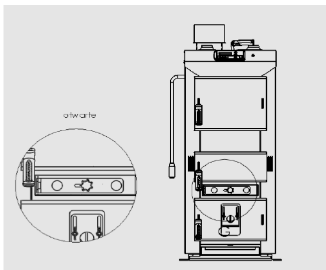
Rys. 10 Regulacja powietrza wtórnego
