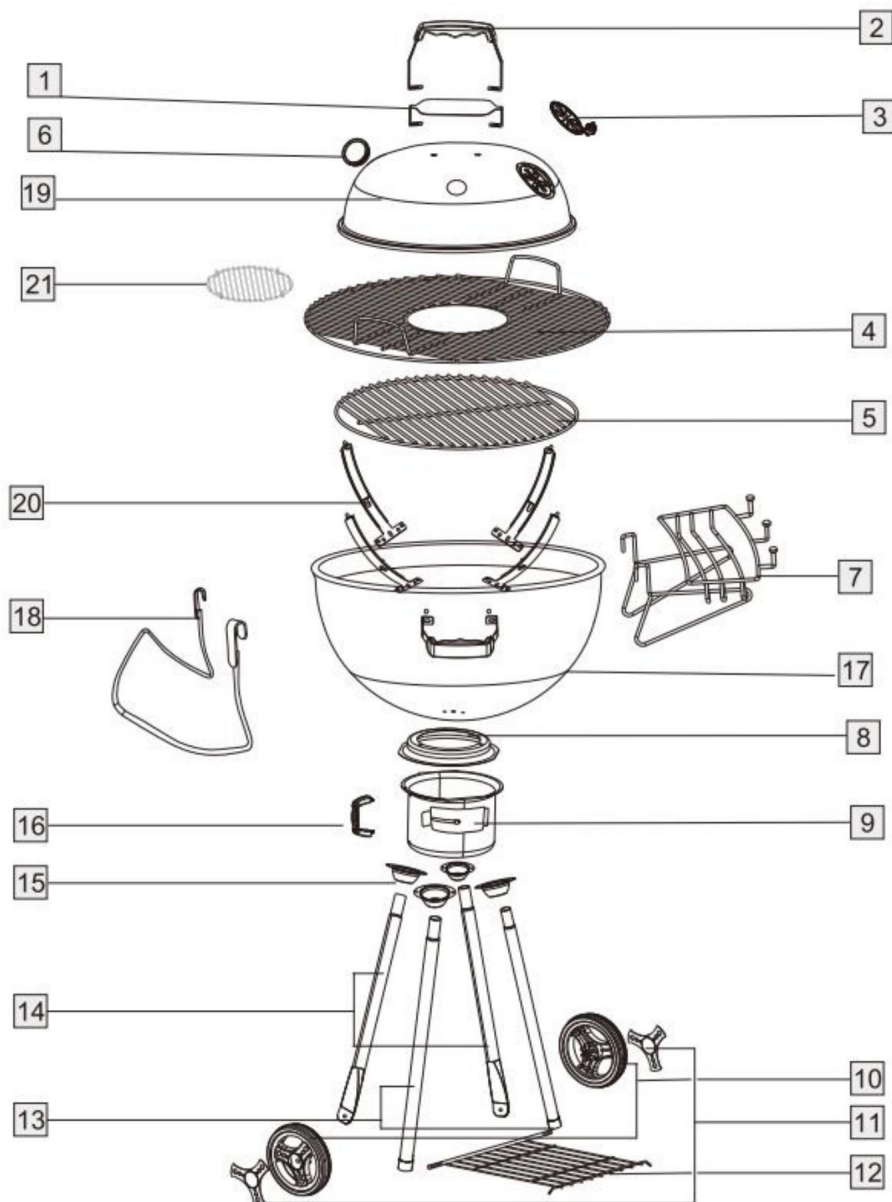
Diagrama de explosión
