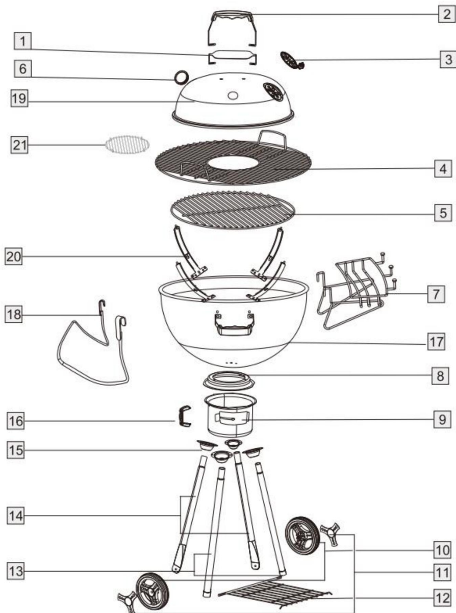
Diagramme d'explosion
