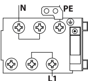
Rys. 2 - Etykieta schematu podłączenia
