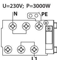
Obr. 2 - Štítek se schématem připojení
