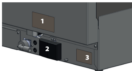
Obr. 3 – 1. Štítek se schématem zapojení; 2. Svorkovnicová skříň; 3. Štítek s údaji o spotřebiči
