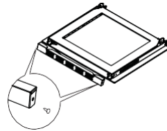
Demontaż wewnętrznego panelu szklanego
