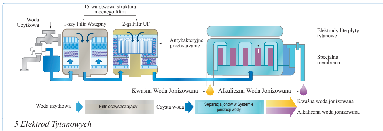
Schemat ukazujący proces wytwarzania wody jonizowanej
