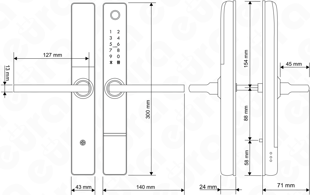
Fig. 3. Dimensioni
