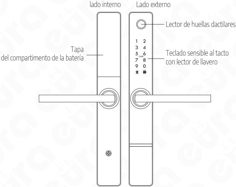
Fig. 2. Construcción
