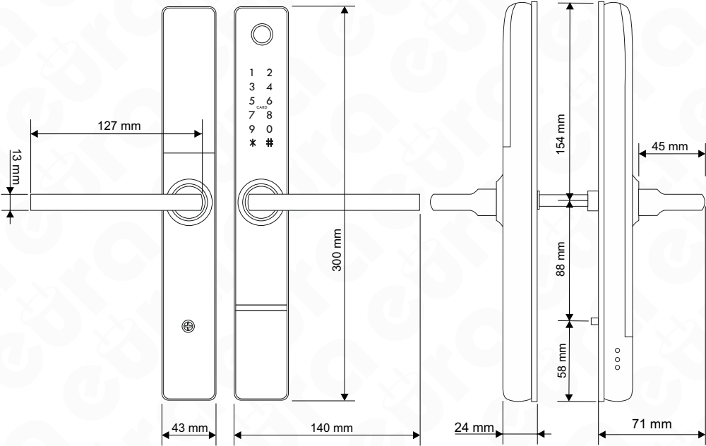
Rys. 3. Wymiary
