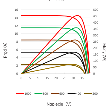
Charakterystyka prądowo - napięciowa (460W)
