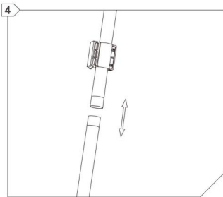
4. Röranslutning.
