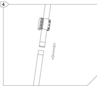
4. Buizenansluiting.
