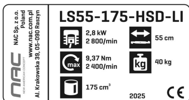
Tabliczka znamionowa
