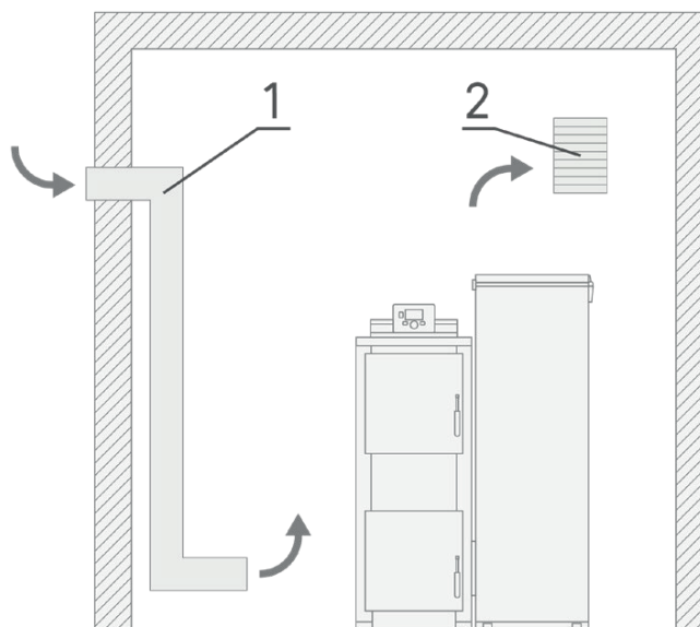
Rys. 7. Ustawienie kotła w kotłowni
