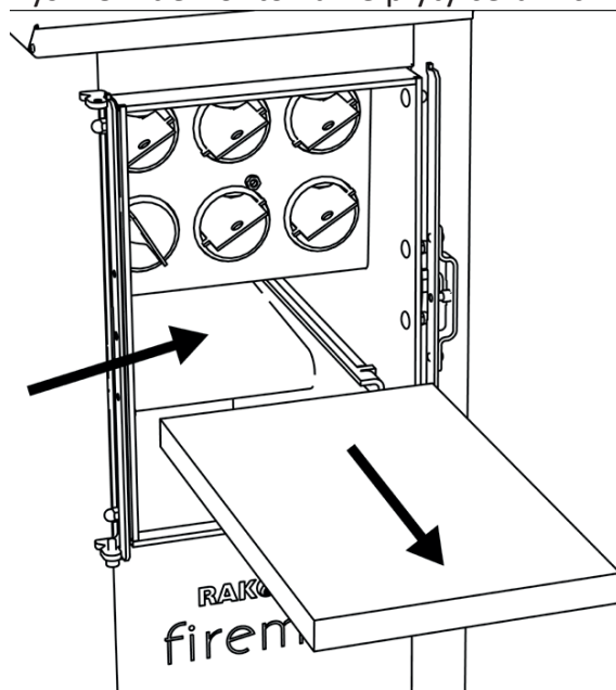
Rys. 13. Zdemontowanie płyty ceramicznej
