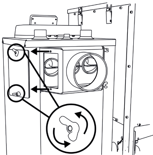
Rys. 15. Oczyszczanie wyczystki czopucha
