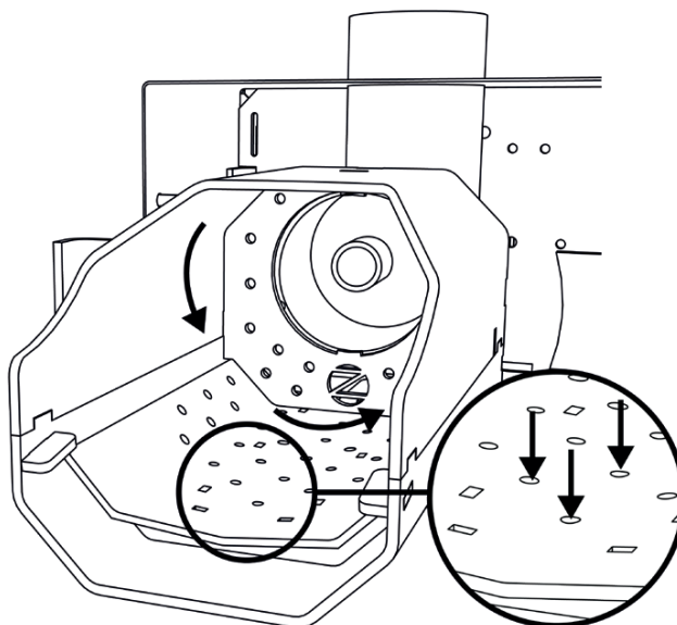
Rys. 20. Czyszczenie rusztu palnika
