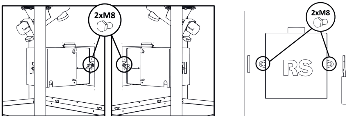
Rys. 18. Odkręcenie śrub mocujących palnik
