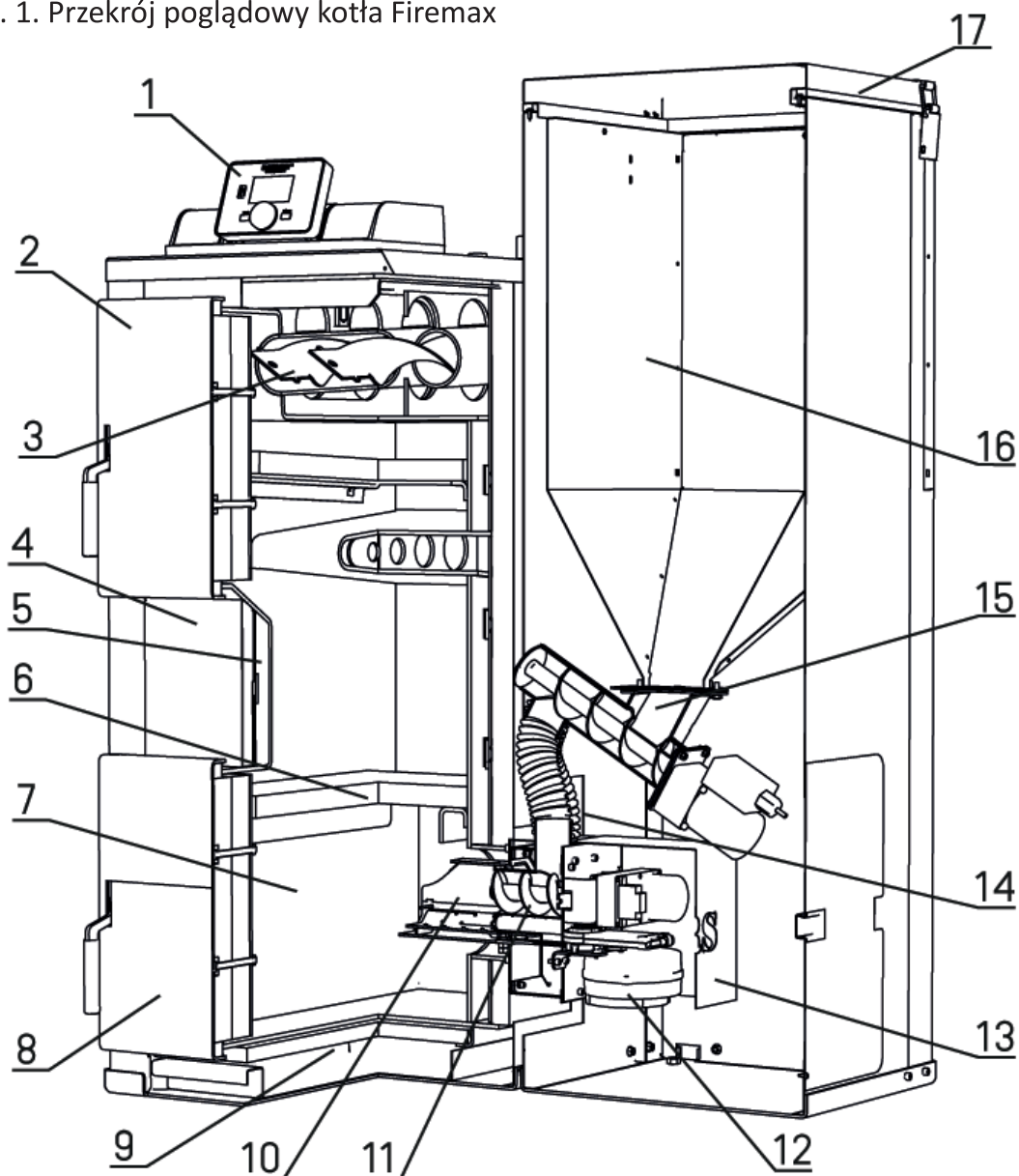
Rys. 1. Przekrój poglądowy kotła Firemax
