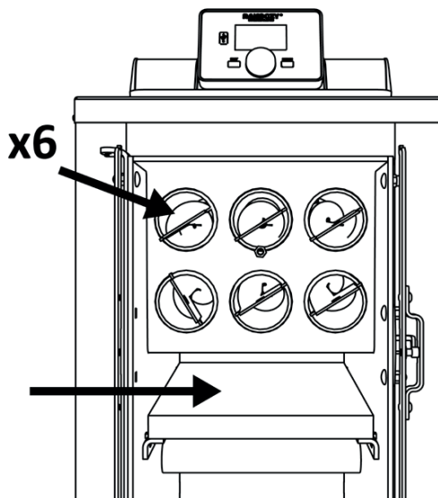
Rys.11. Widok po otwarciu górnych drzwiczek dla kotłów o mocy od 20 do 30kW
