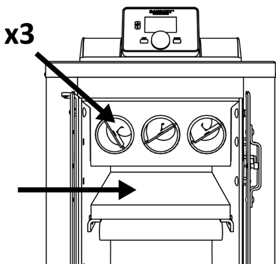
Rys. 10. Widok po otwarciu górnych drzwiczek dla kotłów o mocy 10 i 15kW
