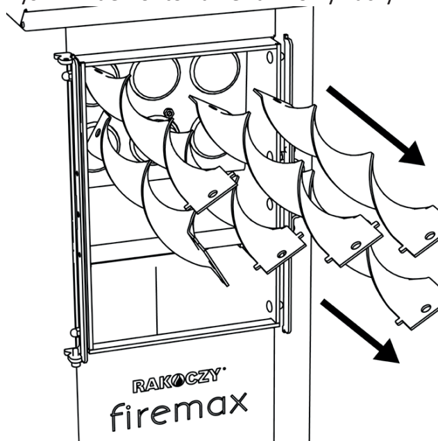
Rys. 12. Zdemontowanie zawirowywaczy
