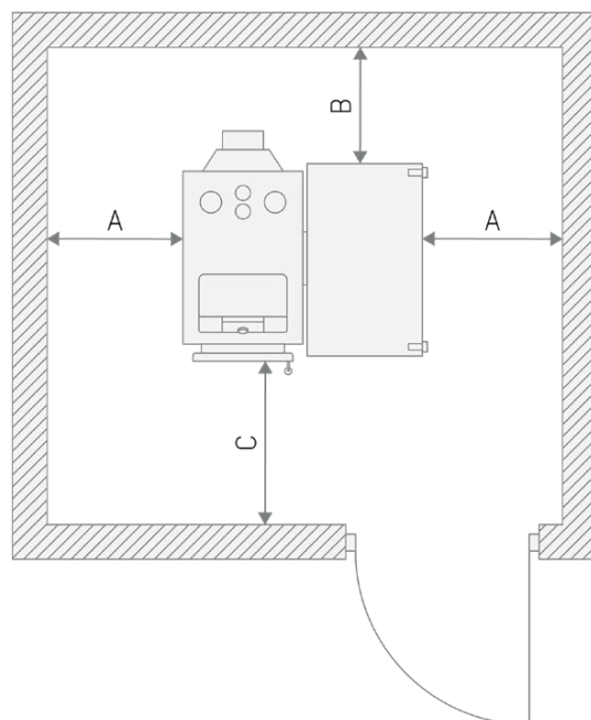
Rys. 8. Ustawienie kotła w kotłowni
