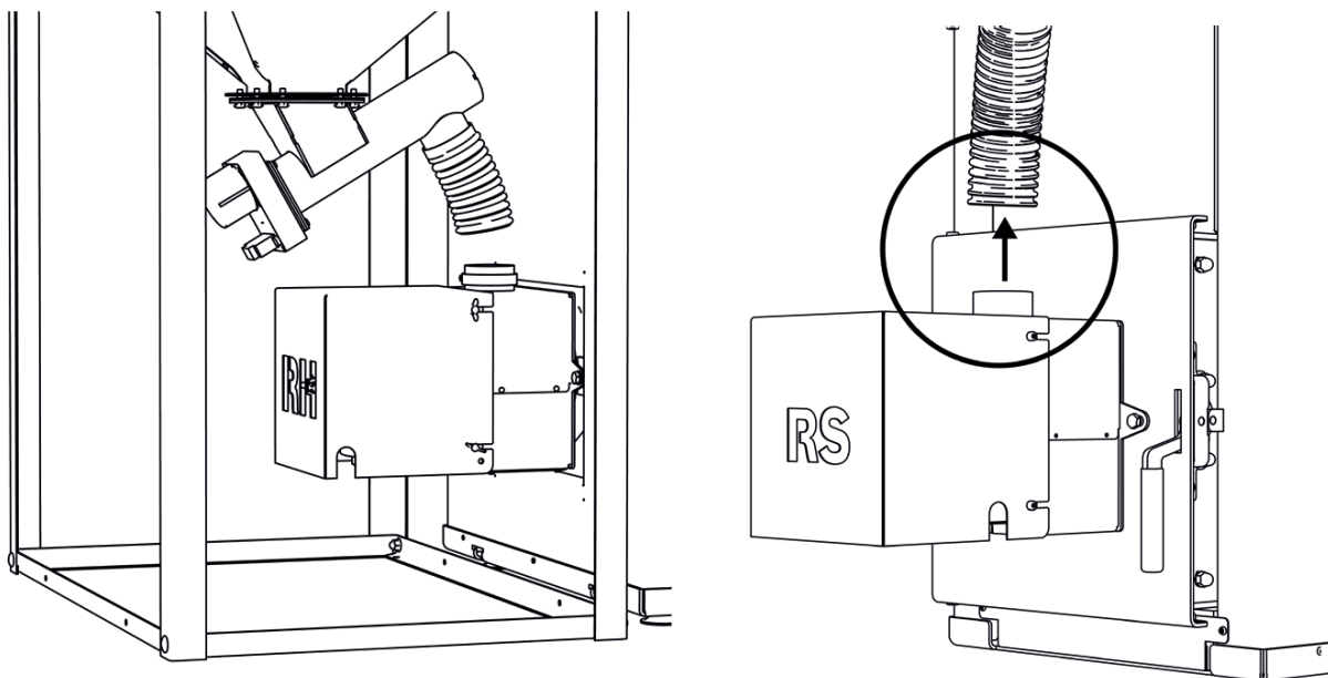
Rys. 17. Demontaż złącza elastycznego
