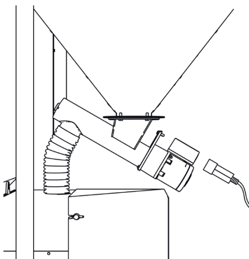
Rys. 16. Odłączenie palnika od zasilania
