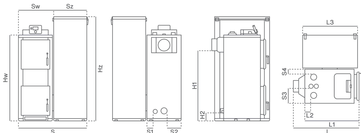
Rys. 3. Wymiary kotła Firemax PLUS
