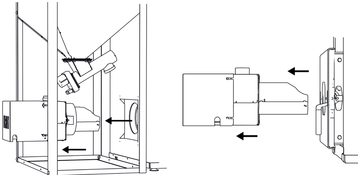
Rys. 19. Wyciąganie palnika
