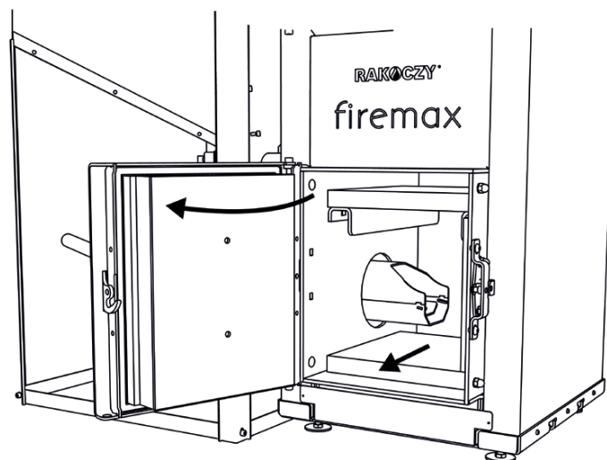
Rys. 14. Opróżnianie popielnika
