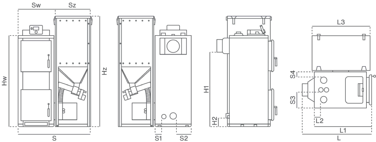
Rys. 4. Wymiary kotła Firemax STANDARD
