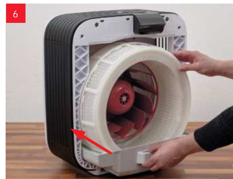
Vaničku na vodu s bubnom nasaďte do prístroja.
