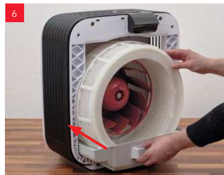
Inserire la vaschetta dell'acqua con il tamburo nell'apparecchio.
