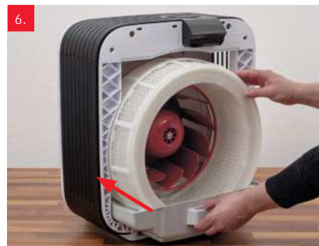
6. Ielieciet ūdens trauku kopā ar trumuli ierīcē.
