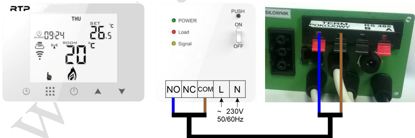
1. Schemat podłączenia termostatu pokojowego.
