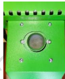
Fot.6. Okresowo czyścić wlot peletu do palnika.
