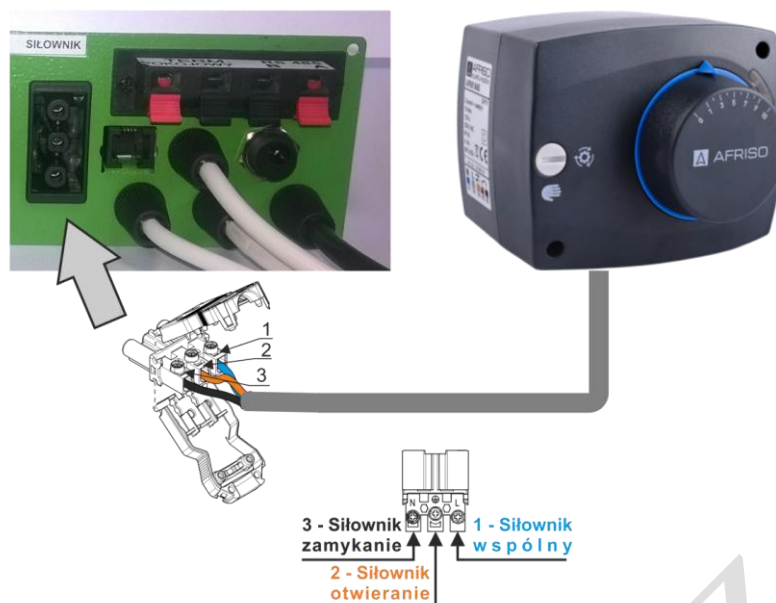
2. Schemat podłączenia siłownika zaworu mieszającego.
