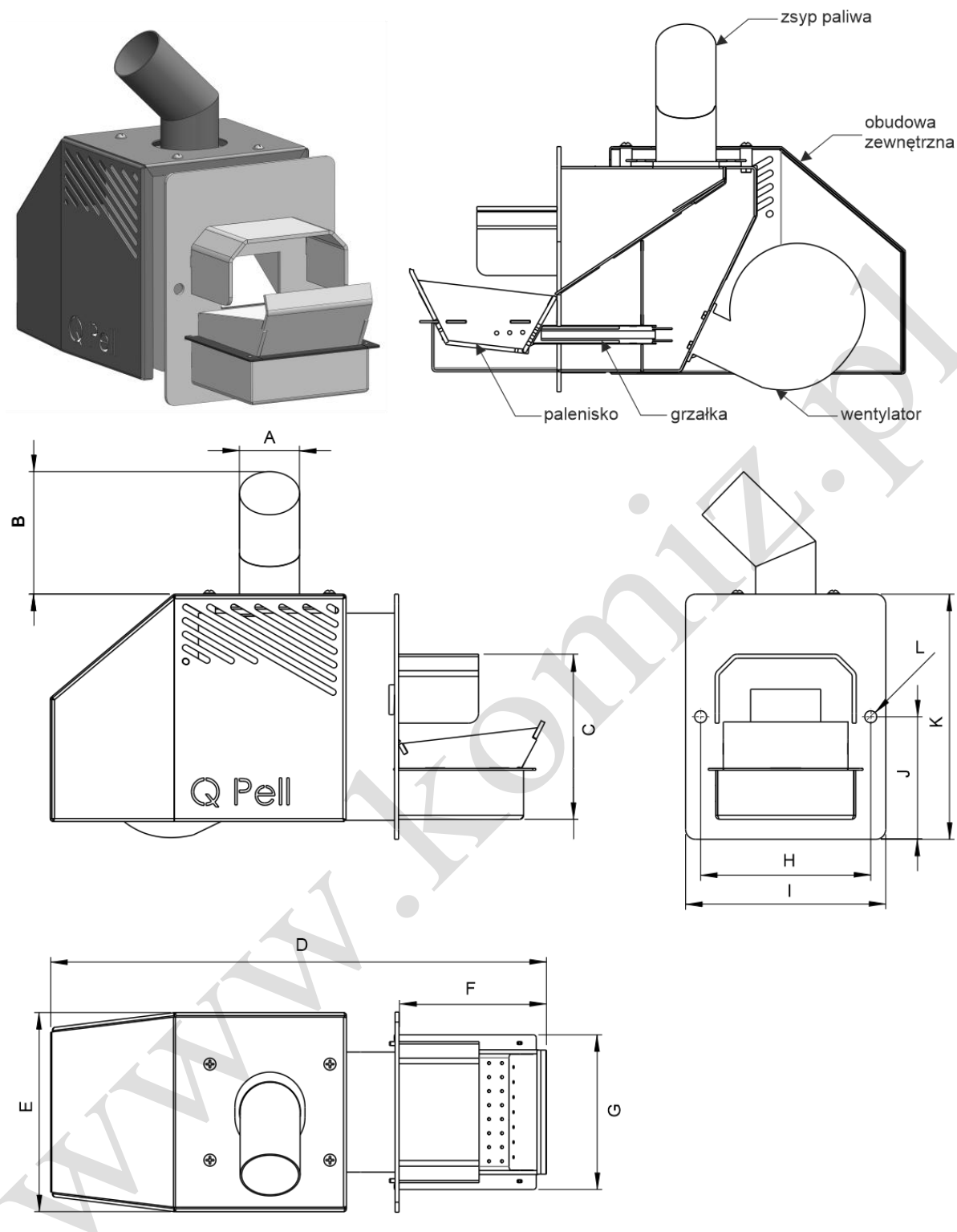
Rys.3.1.2.Wymiary palnika QPell 8 – 24 kW.
