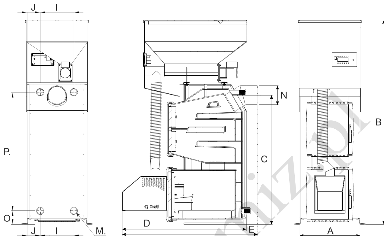
Rys.3.2.2.Wymiary kotłów sztoker ® bio 8 – 12 G.
