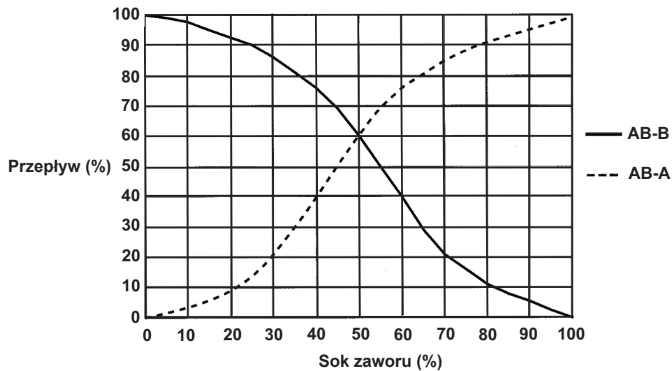
Rys. 9 Typowa charakterystyka przełączania zaworu 3-drogowego przy stałym ciśnieniu na wejściu AB
