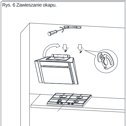
Rys. 6 Zawieszanie okapu.
