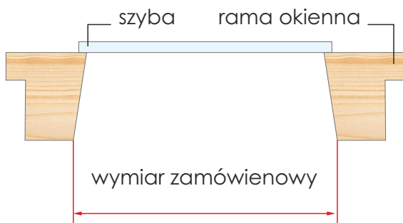
Przekrój okna ze skosem
