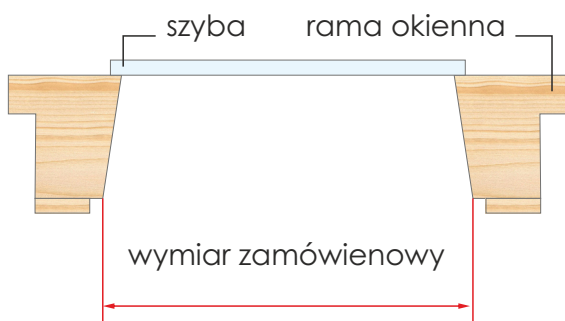
Przekrój okna Velux
