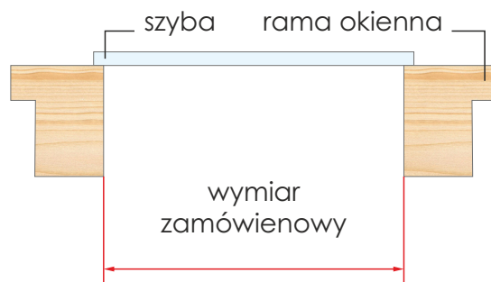
Przekrój okna prostego
