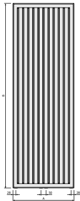
Vertical, typy 20, 21, 22, widok z przodu
