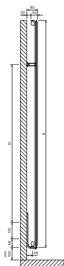
Nowy Vertical, typ 10, widok z boku
