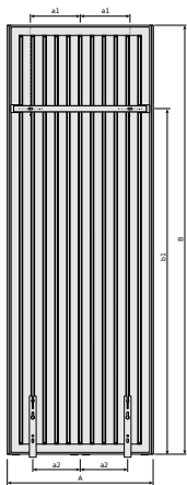
Vertical, zawieszenia MCW6, widok od tyłu
