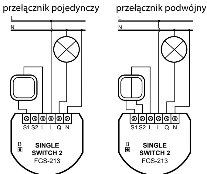
Schematy podłączenia - Single Switch 2
