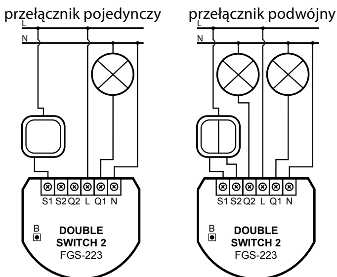
Schematy podłączenia - Double Switch 2
