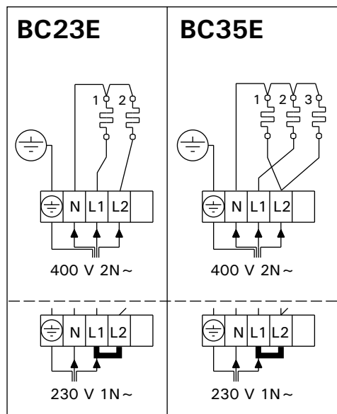
Rys. 10. Schemat elektryczny (BC-E) Obrázek 10. Zapojení topného tělesa BC-E
