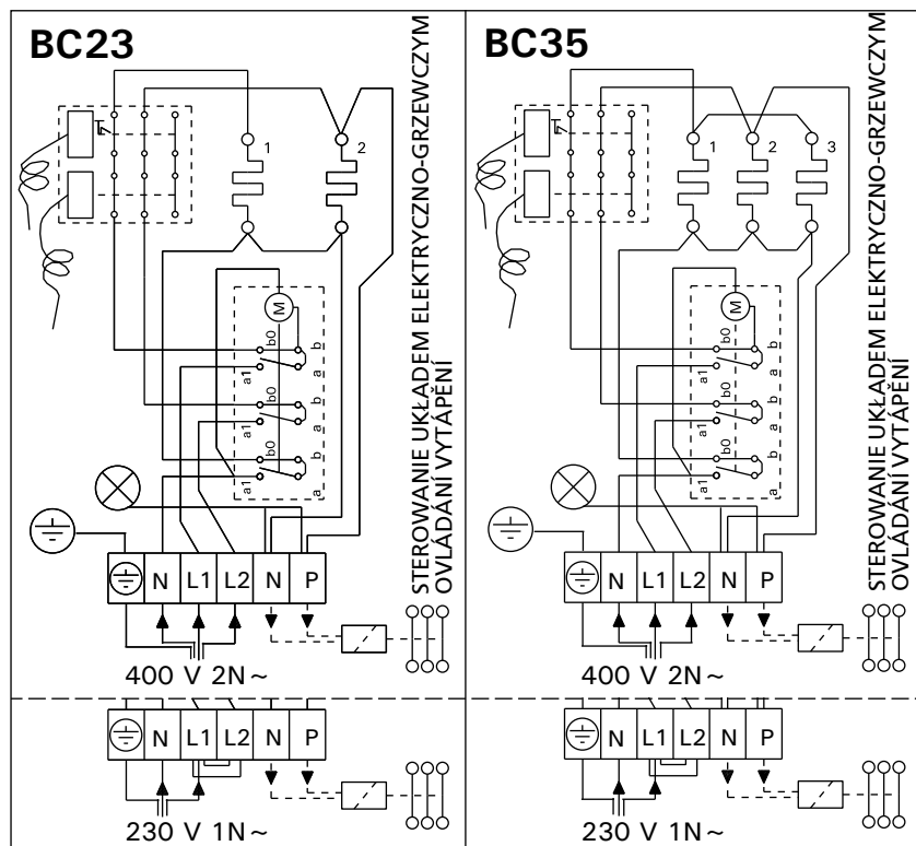
Rys. 9. Schemat elektryczny (BC) Obrázek 9. Zapojení topného tělesa BC
