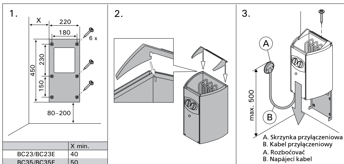
Rys. 7. Mocowanie pieca na ścianie (wymiały w milimetrach)
