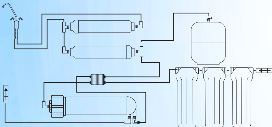
SCHEMAT INSTALACJI:
