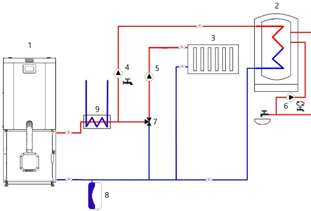
Rysunek 18 - Schemat obiegu C.W.U. i C.O. układ zamknięty z węzownicą schładzającą. 1 - kocioł, 2 – wymiennik C.W.U., 3 – grzejniki C.O., 4 -pompa obiegowa C.W.U., 5 – pompa obiegowa C.O., 6 – pompa cyrkulacyjna, 7 – trójdrożny zawór mieszający, 8 – przeponowe naczynie wzbiorcze, 9 – węzownica schładzająca.
