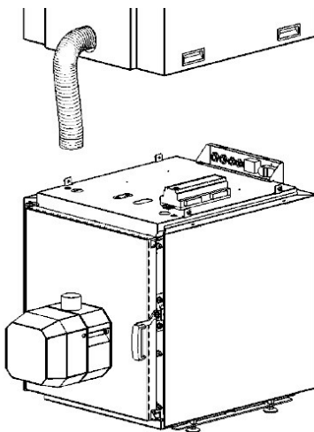
Rysunek 20 - Umiejscowienie sterownika i dławików
