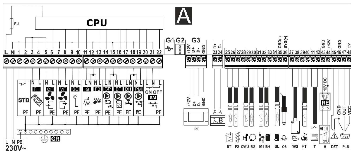
Rysunek 22 - Schemat połączeń elektrycznych regulatora L N PE -zasilanie sieciowe 230V ~, CPU - sterowanie, FU – bezpiecznik, STB -wejście do ogranicznika temperatury bezpieczeństwa, FH – podajnik główny CF – wentylator nadmuchowy palnika, VF – wentylator wyciągowy, SC – silnik obrotowy czyszczenia palnika, IG – zapalarka, FB – podajnik palnika, CP – pompa cyrkulacji CWU, BP -pompa kotła, DH -pompa CWU, PM – pompa mieszacza 1, SM – siłownik mieszacza 1, RT – panel pokojowy ecoSTER TOUCH z funkcją termostatu pokojowego, λ – moduł sondy Lambda, B – moduł do obsługi dodatkowych obiegów grzewczych, BT – czujnik temperatury kotła typu CT4, FS – czujnik temperatury podajnika typu CT4, CWU -czujnik temperatury CWU typu CT4, RS – czujnik temperatury wody powracającej do kotła typu CT4, M1 -czujnik temperatury obiegu regulowanego (mieszacza 1) typu CT4, BH – czujnik temperatury bufora górny typu CT4, BL - czujnik temperatury bufora dolny typu CT4, OS – optyczny czujnik jasności płomienia, WS – pogogowy czujnik temperatury typu CT6-P, FT – czujnik temperatury spalin typu CT2S, T -termostat pokojowy (zwierno-rozwierny), H – wyjście napięciowe do sterowania kotłem rezerwowym R lub do sygnalizacji alarmów AL , RELAY – przekaźnik 12VDC, DZT – czujnik otwarcia drzwi kotła lub klapy zasobnika, PLS – czujnik poziomu paliwa
