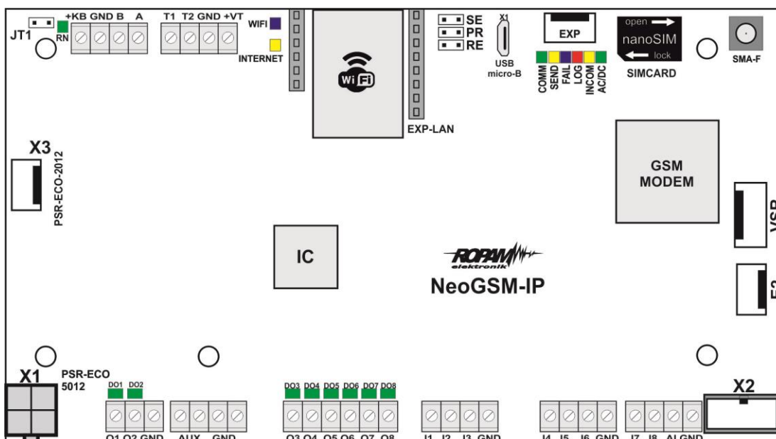
Widok: NeoGSM-IP PCB.
