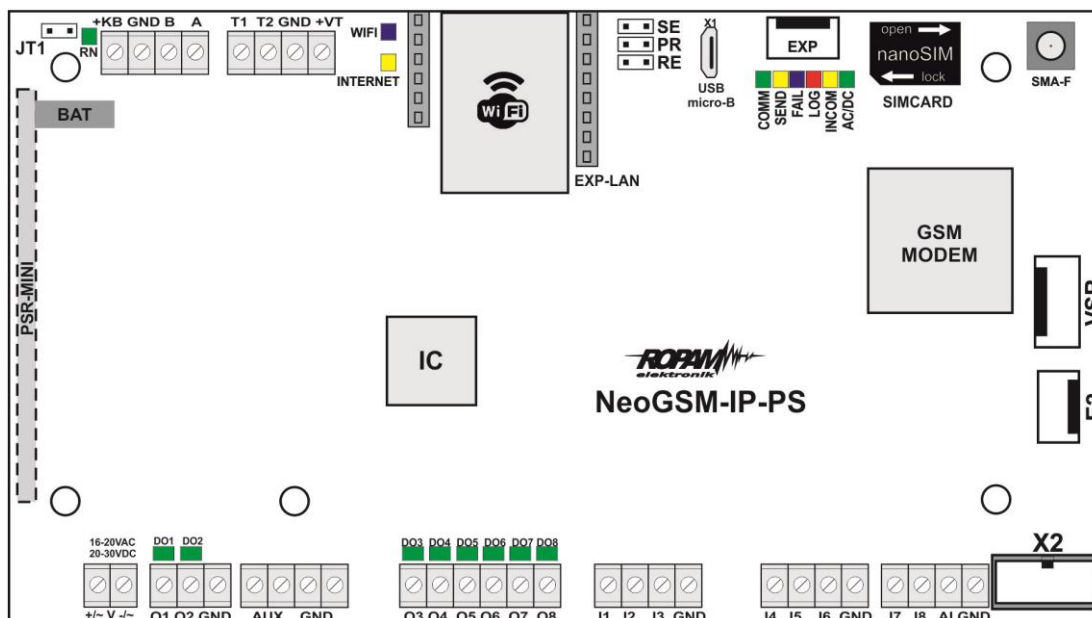
Widok: NeoGSM-IP-PS PCB.
