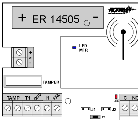
Widok modułu IO-Aero
