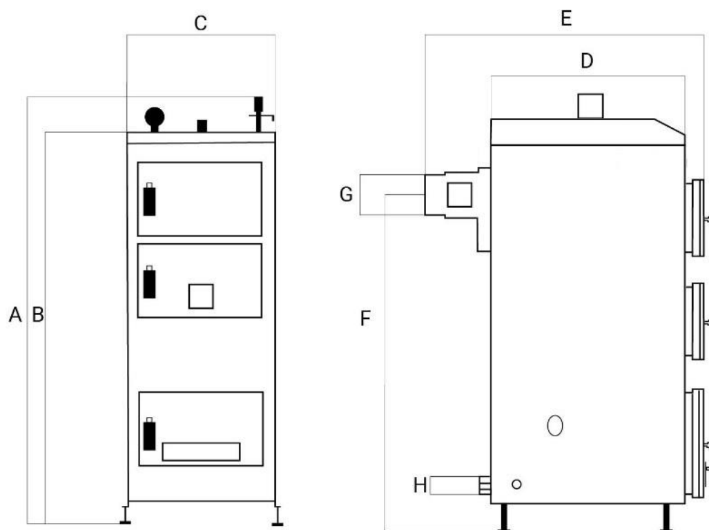
Rysunek 2. Wymiary kotła EKO UKS PLUS (w cm).
